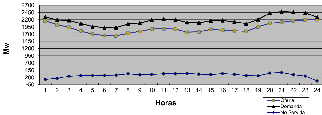
Evolución de la Generación en las 24 Hrs del 15 de junio de 2017
