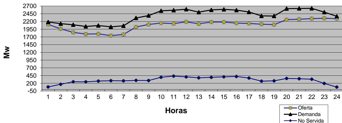
Evolución de la Generación en las 24 Hrs del 27 de junio de 2017
