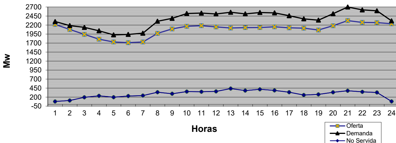
Evolución de la Generación en las 24 Hrs del 25 de julio de 2017
