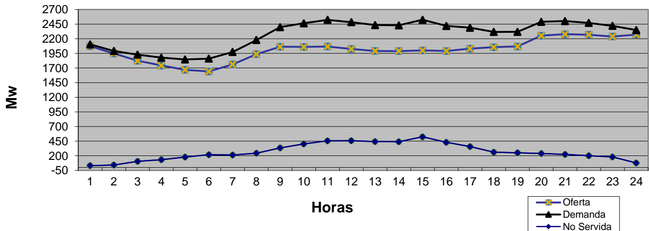
Evolución de la Generación en las 24 Hrs del 17 de julio de 2017
