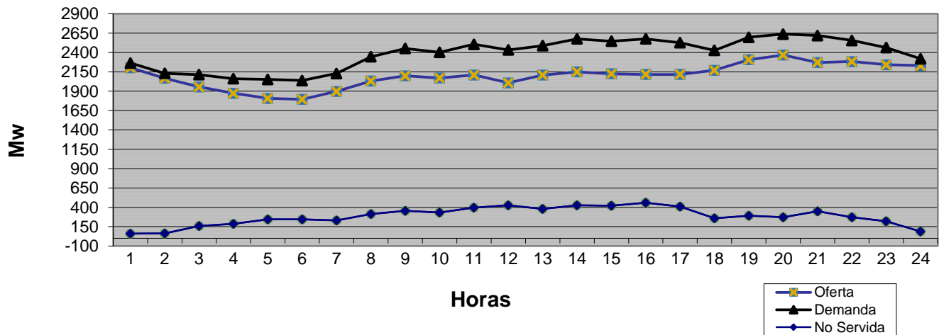
Evolución de la Generación en las 24 Hrs del 16 de octubre de 2017
