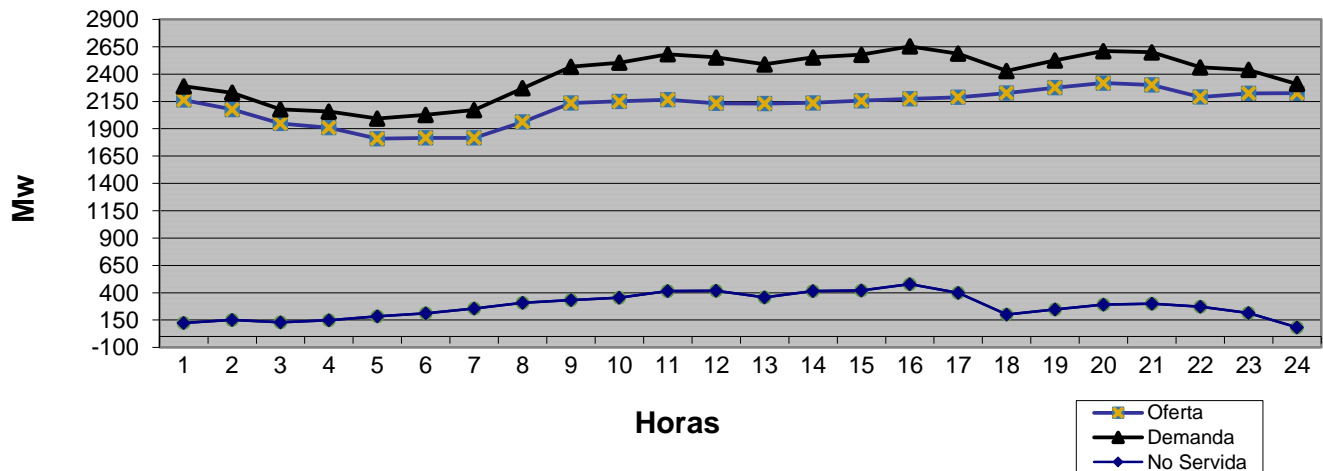
Evolución de la Generación en las 24 Hrs del 02 de octubre de 2017
