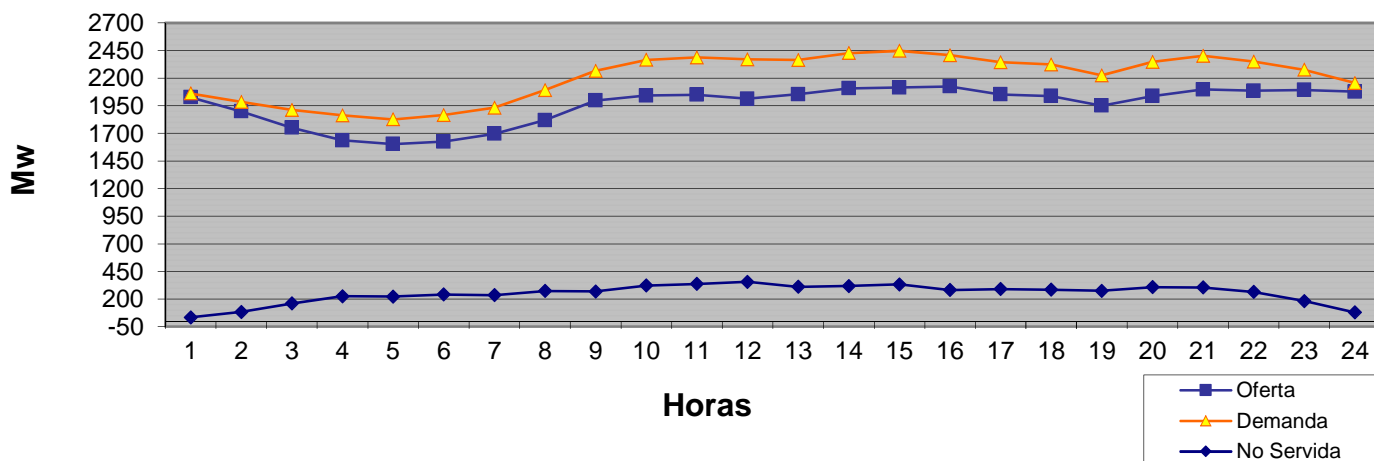
Evolución de la Generación en 24 Hrs del 26 de Octubre 2016
