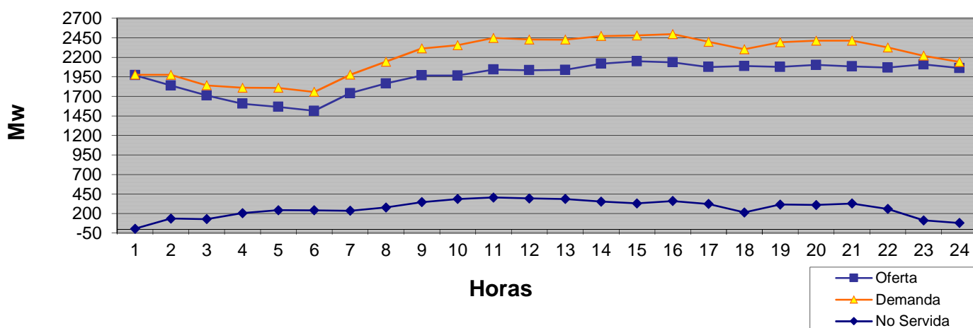
Evolución de la Generación en 24 Hrs del 24 de Octubre 2016
