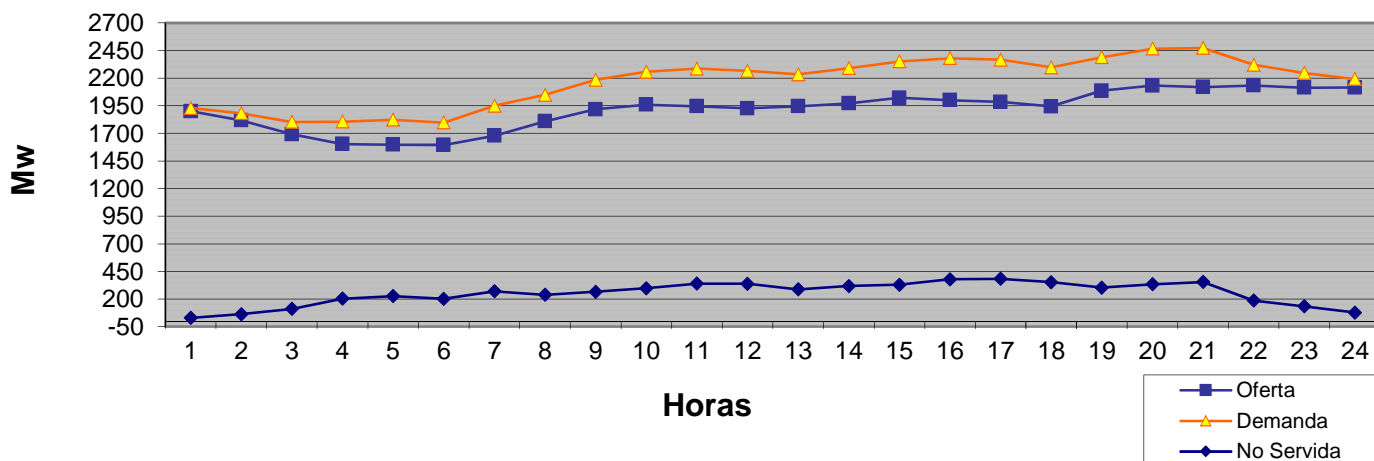
Evolución de la Generación en 24 Hrs del 02 de Noviembre 2016
