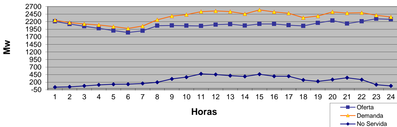
Evolución de la Generación en 24 Hrs del 14 de julio 2016
