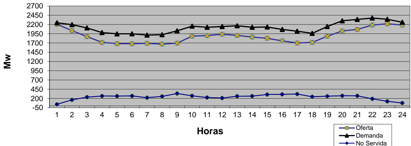
Evolución de la Generación en las 24 Hrs del 20 de agosto de 2017
