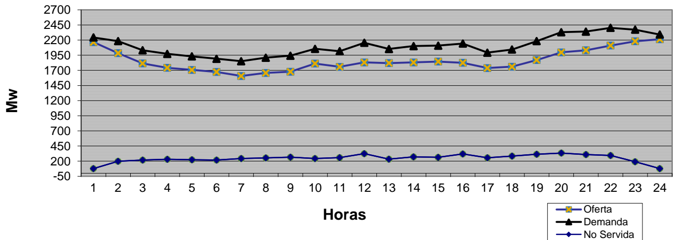
Evolución de la Generación en las 24 Hrs del 13 de agosto de 2017
