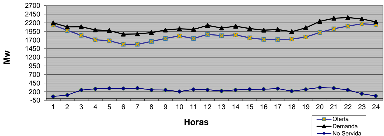
Evolución de la Generación en las 24 Hrs del 06 de agosto de 2017
