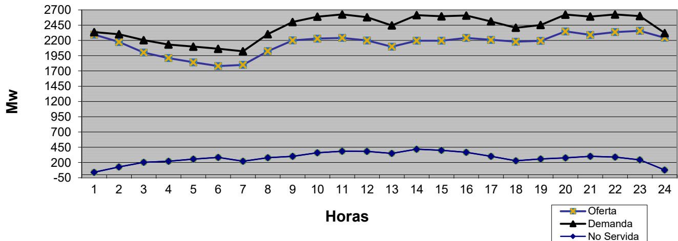
Evolución de la Generación en las 24 Hrs del 01 de agosto de 2017
