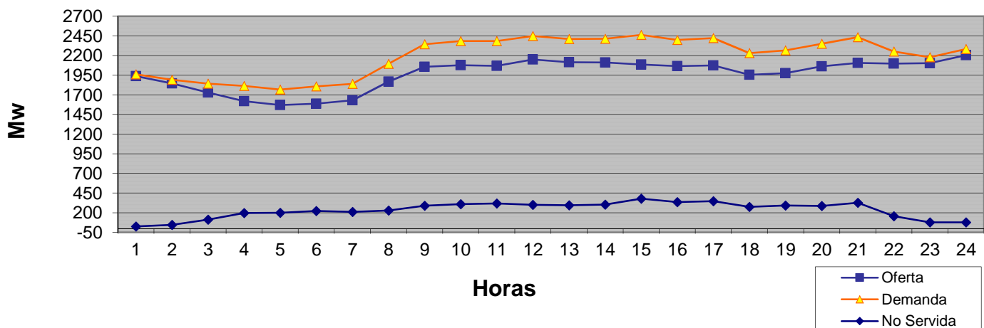
Evolución de la Generación en 24 Hrs del 12 de agosto 2016
