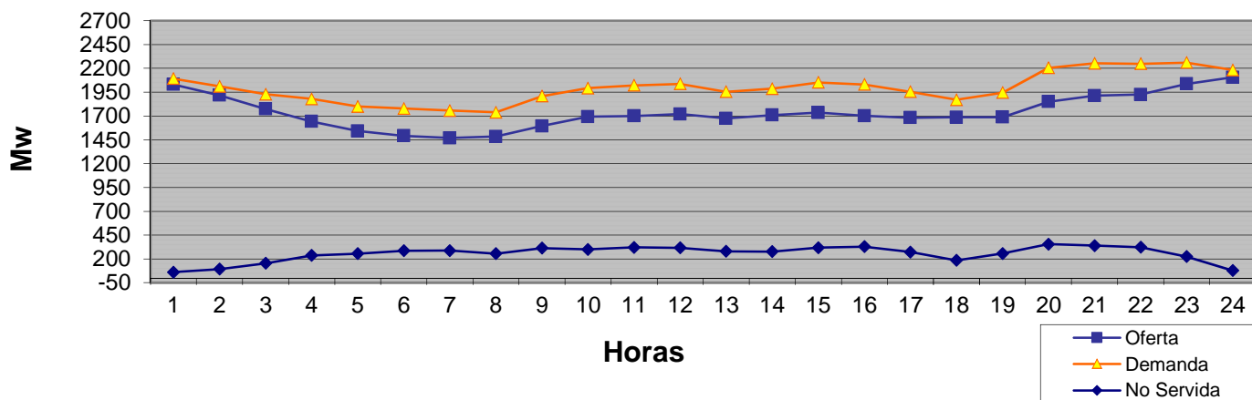
Evolución de la Generación en 24 Hrs del 26 de junio 2016
