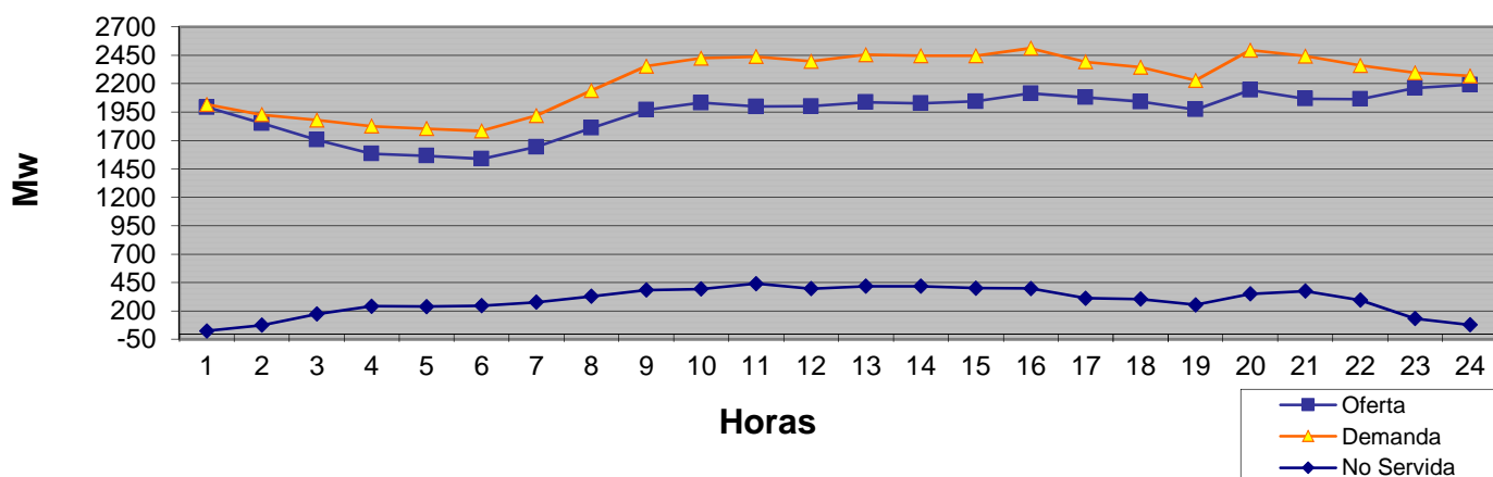
Evolución de la Generación en 24 Hrs del 23 de junio 2016
