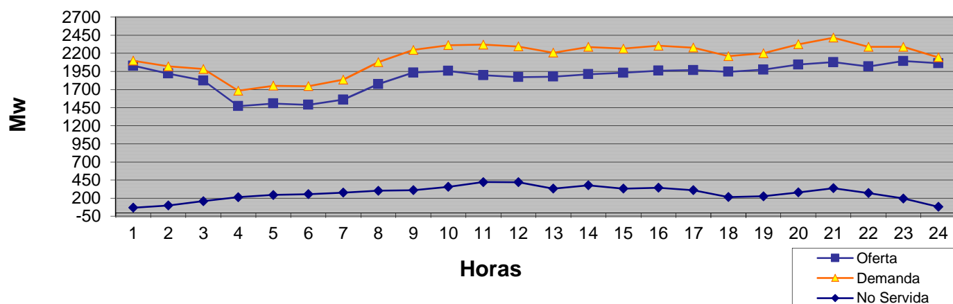
Evolución de la Generación en 24 Hrs del 21 de junio 2016
